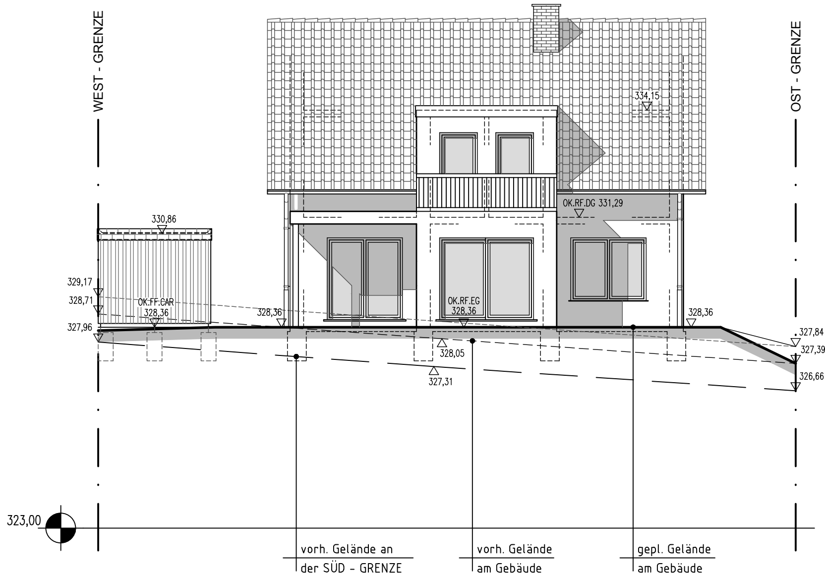
SÜDANSICHT
